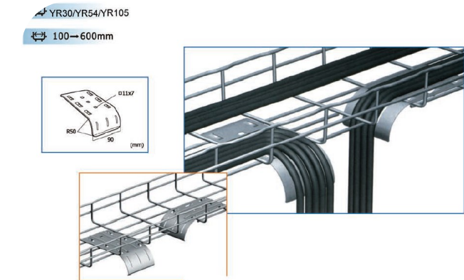
Guías para desviación de cables.
