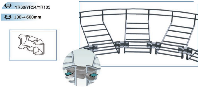
Sujetadores para curvas.
