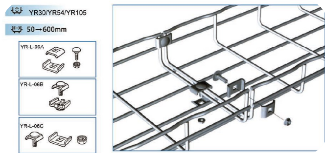
Sujetadores universal empernado.
