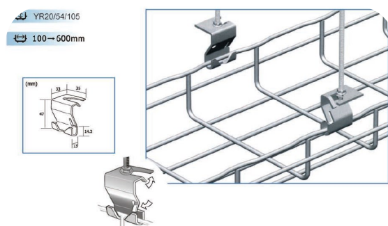
Soportes lateral de anclaje superior.
