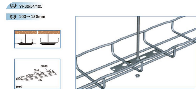
Soportes central de anclaje superior.
